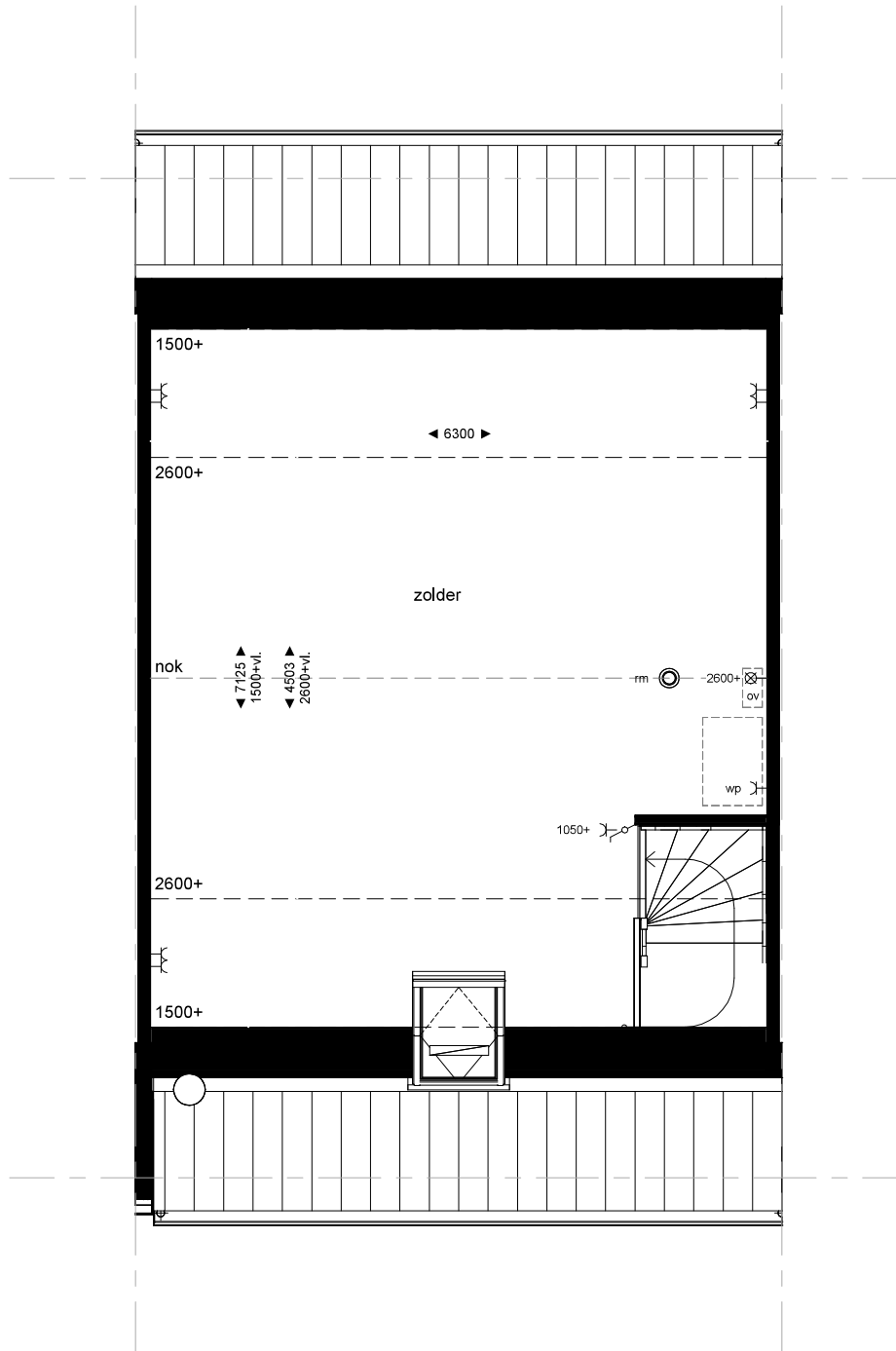
1e verdieping 1 : 50
